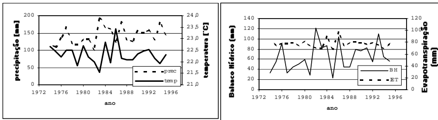
Fig. 4. Média mensal aritmética do período de vegetação (outubro até abril) dos dados originais da temperatura e precipitação (esquerda) e do balanço hídrico (BH) e índice de evapotranspiração (IET)(direita).
